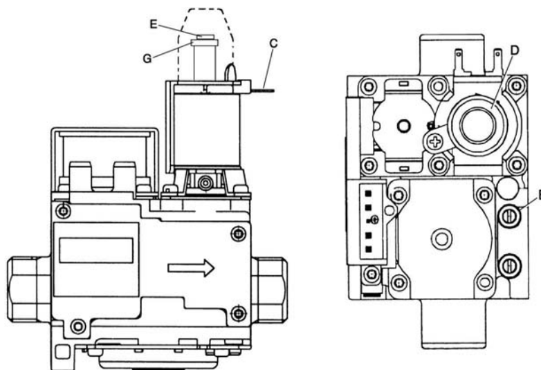
рис. 10 - Газовый клапан
