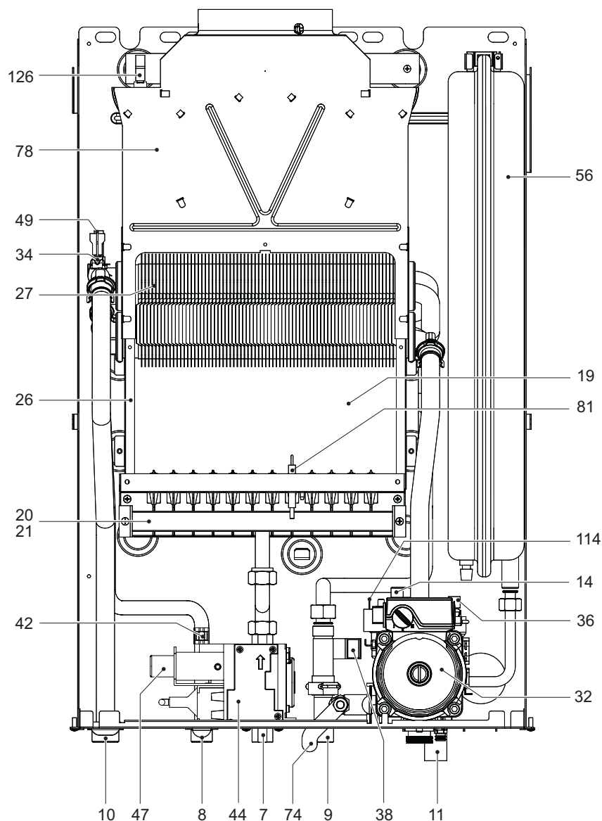
рис. 13 - Общий вид
