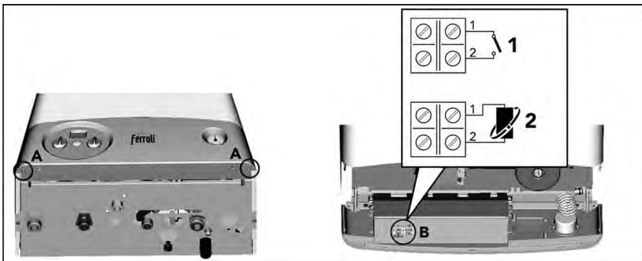
рис. 8 - Доступ к клеммной коробке
