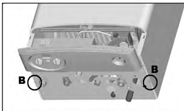
рис. 11 - Снятие кожуха
