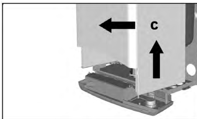
рис. 11 - Снятие кожуха
