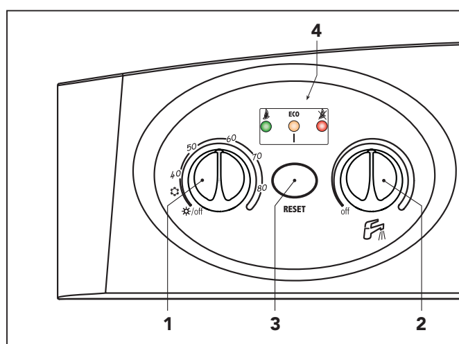
рис. 1 - Панель управления
