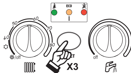
рис. 9 - Режим TEST
