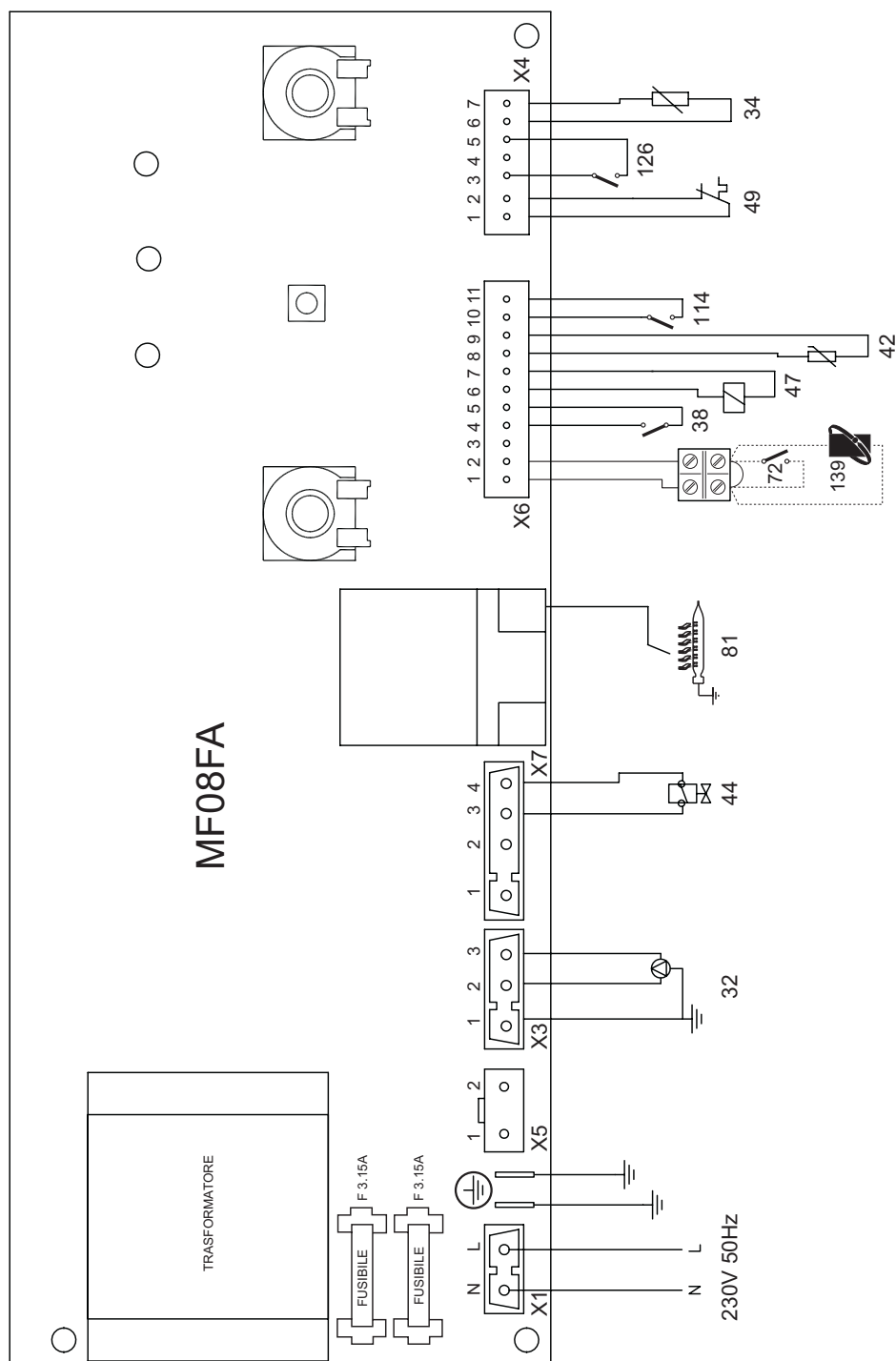
рис. 15 - Электрическая схема
