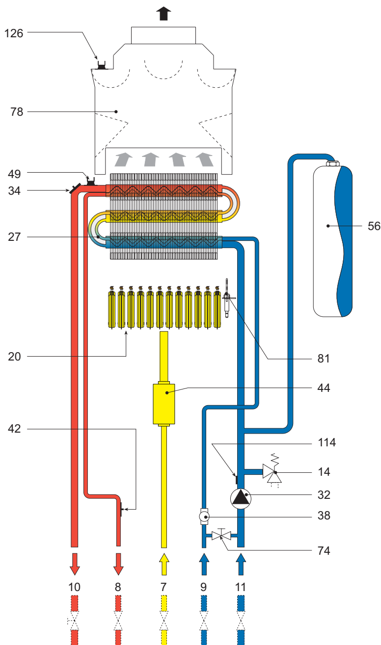
рис. 14 - Схема системы отопления и контура ГВС
