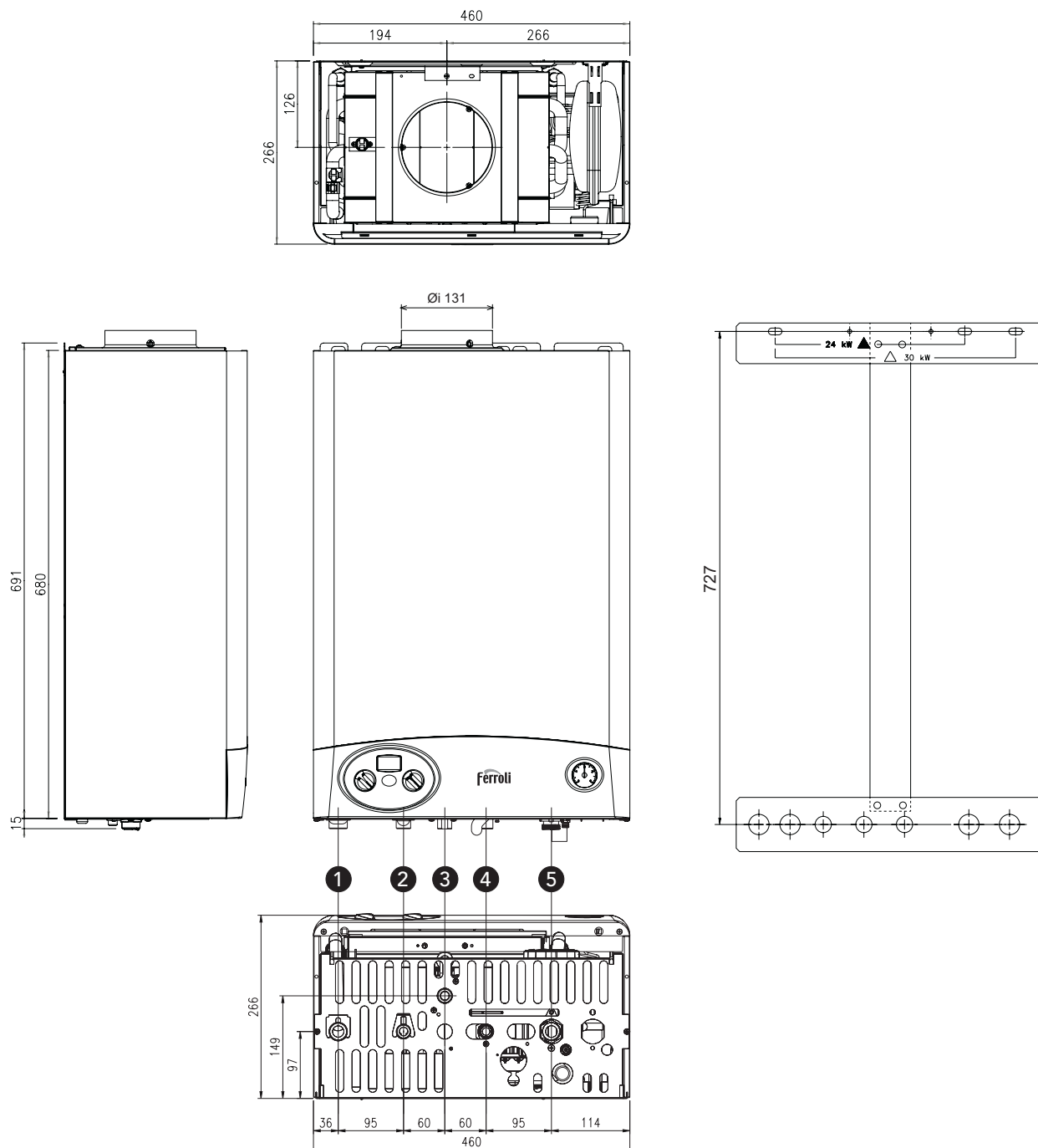
рис. 12 - Габаритные размеры и подключения
